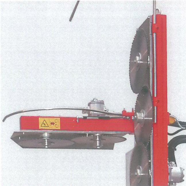
GÓRNY ZESPÓŁ TNĄCY REGULOWANY pod względem wysokości, z manualną suwnicą
